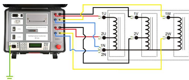
Branchement de TRT03 à un autotransformateur triphasé
