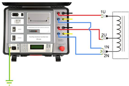
Branchement de TRT03 à un autotransformateur monophasé
