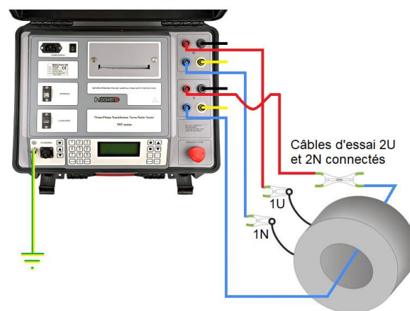
Branchement de TRT03 à un transformateur de courant démonté
