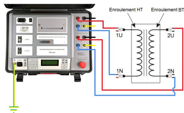
Branchement de TRT03 à un transformateur monophasé
