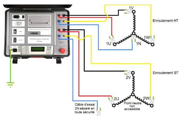
Branchement de TRT03 à un transformateur triphasé
