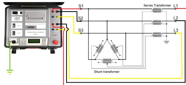
Branchement de TRT3x à un transformateur déphaseur
