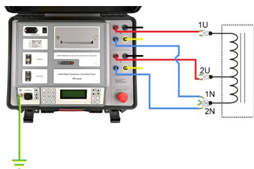
Branchement de TRT3x à un autotransformateur monophasé
