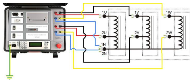
Branchement de TRT3x à un autotransformateur triphasé
