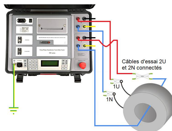
Branchement de TRT3x à un transformateur de courant démonté
