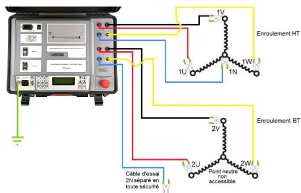
Branchement de TRT3x à un transformateur triphasé
