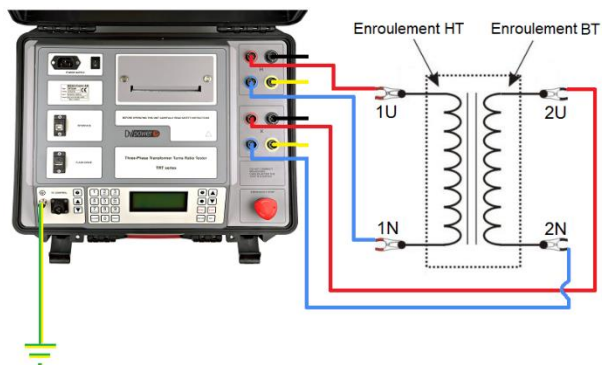
Branchement de TRT3x à un transformateur monophasé
